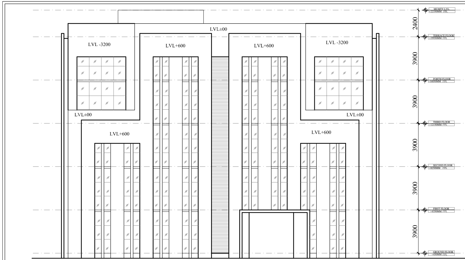
ELEVATION-A
